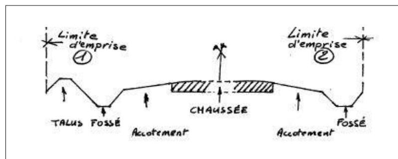
Profil en travers type
