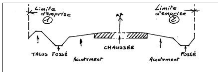
Profil en travers type
