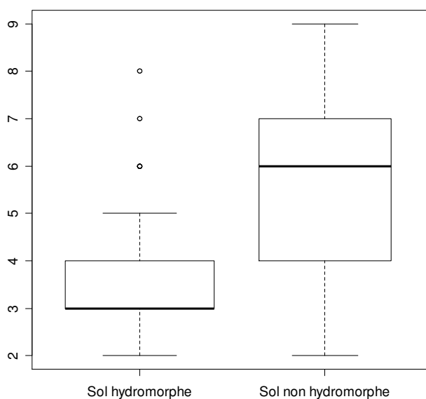
Figure 34 : niveau hydrique bio-indiqué vs. hydromorphie. L'axe du niveau hydrique est gradué du pôle hygrophile (1) au pôle xérophile (9, annexe 10.3).
